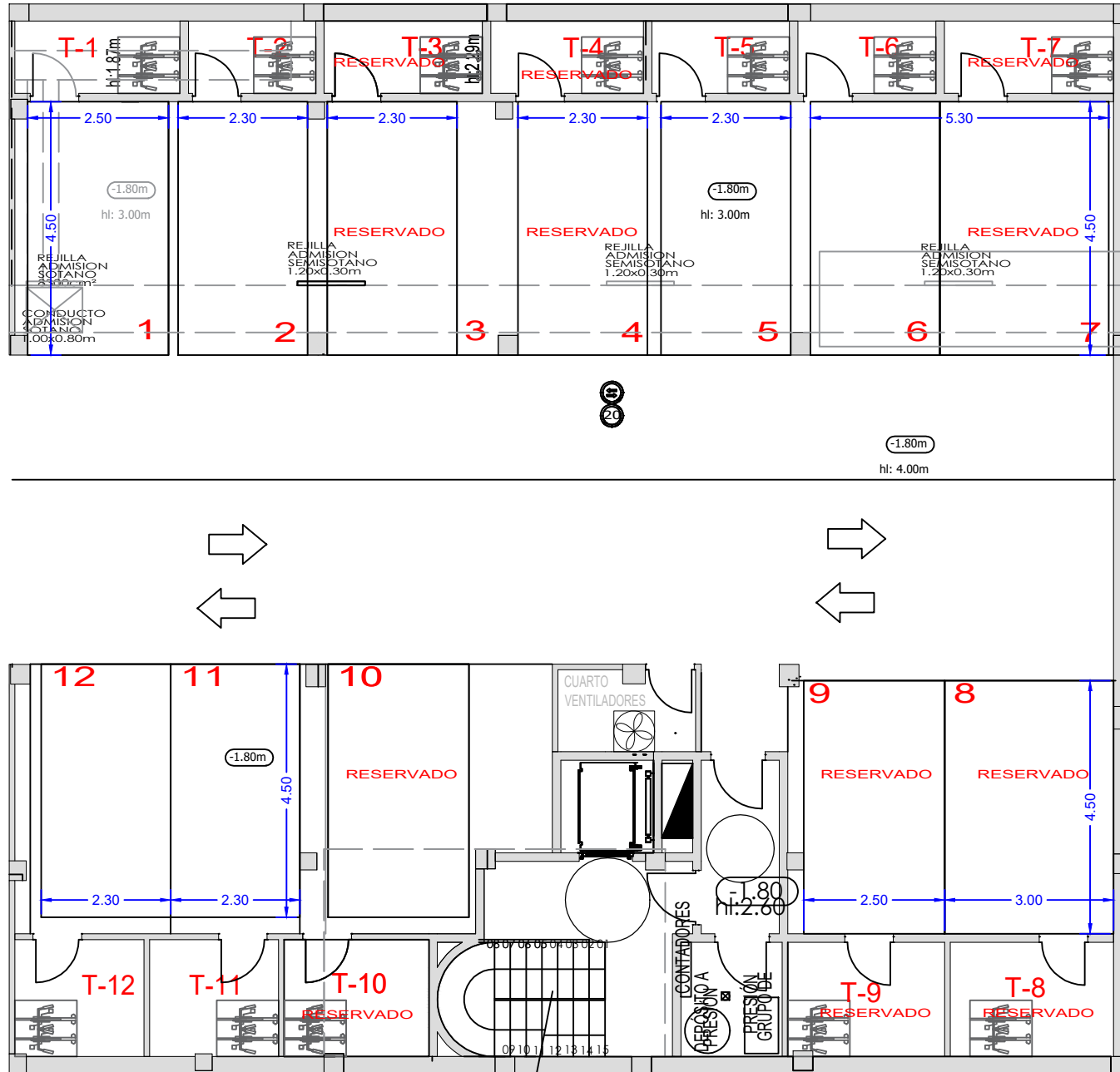
PLANTA SEMISÓTANO
