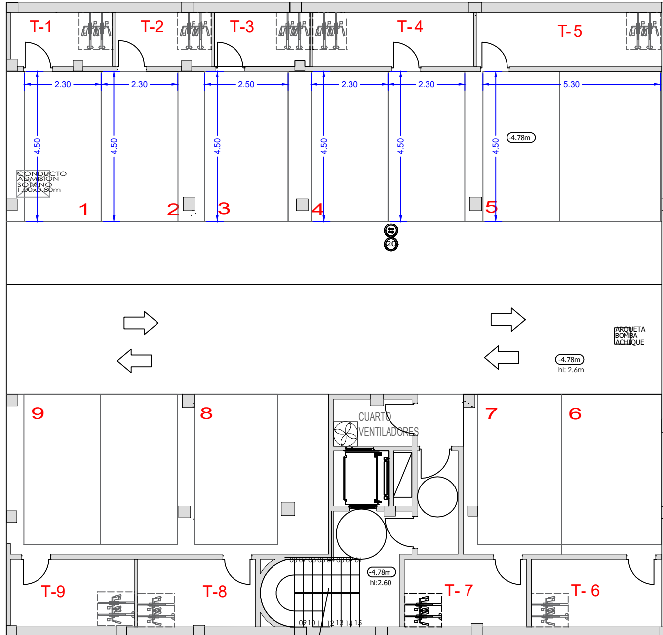
PLANTA SÓTANO
